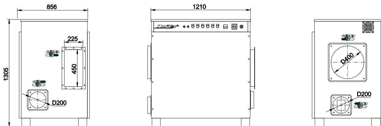
Рис 2. Размеры осушителя воздуха AD-3000
